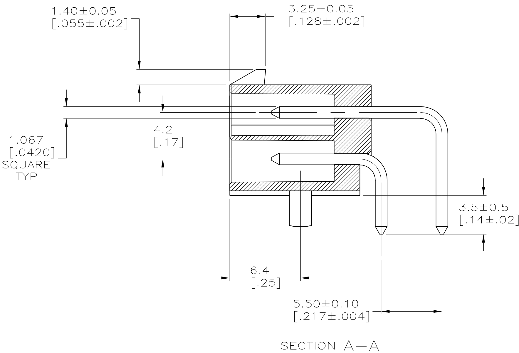
SECTION A-A
