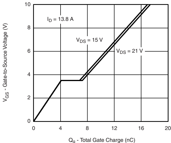
I_D = 13.8\text{ A} V_{DS} = 15\text{ V} V_{DS} = 21\text{ V} Gate Charge
